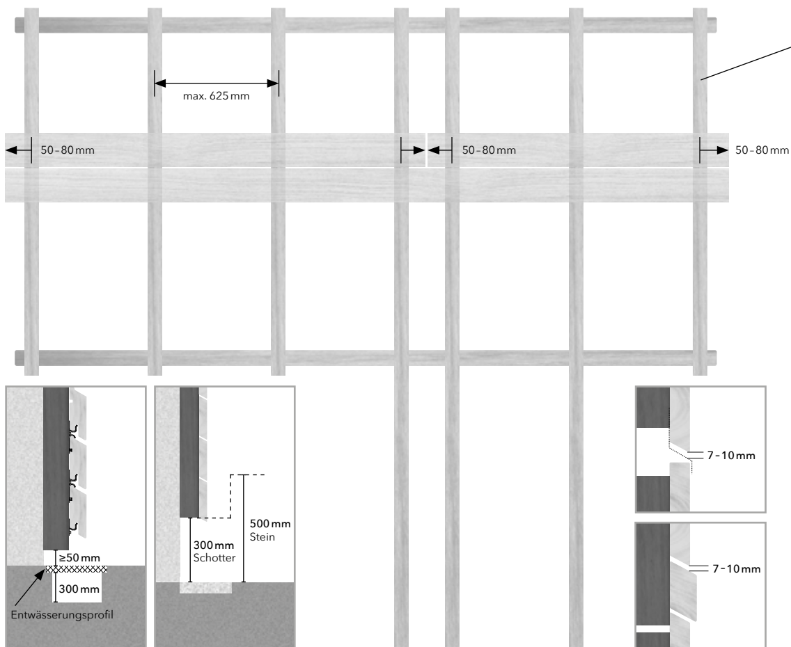
Spritzwasserschutz im Sockelbereich
