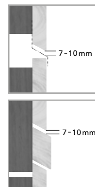
Vertikale Stoßfuge
